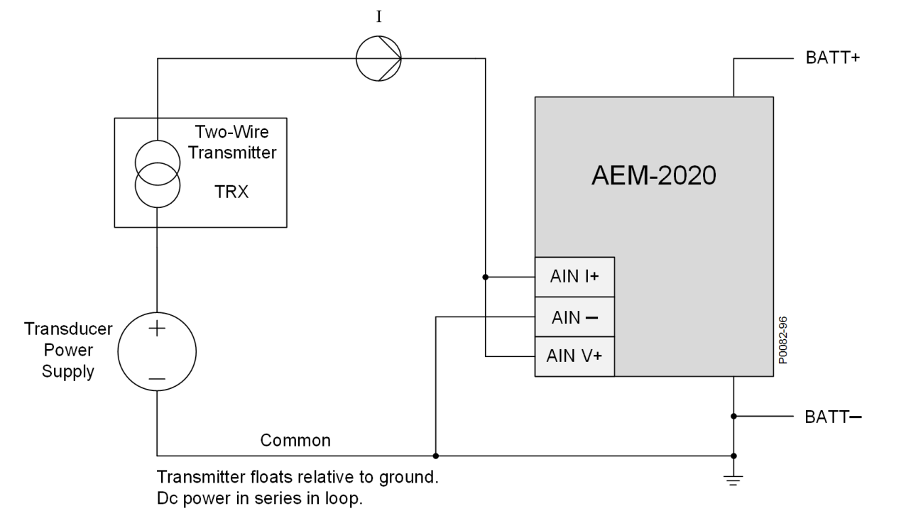
图 11-4. 模拟量输入 - 电流输入接线，II 型 2 线电路
