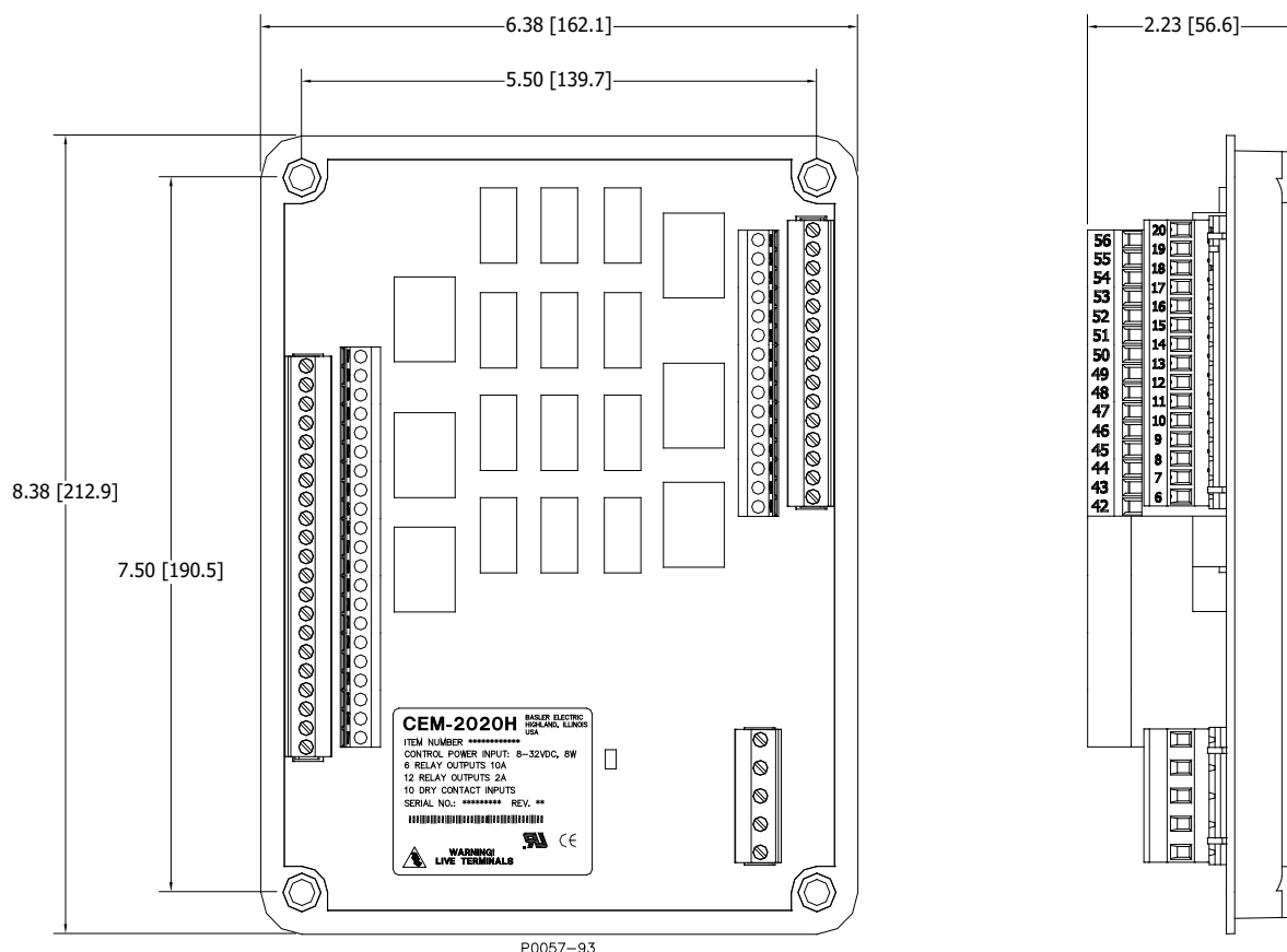
图 10-2. CEM-2020H 总尺寸
