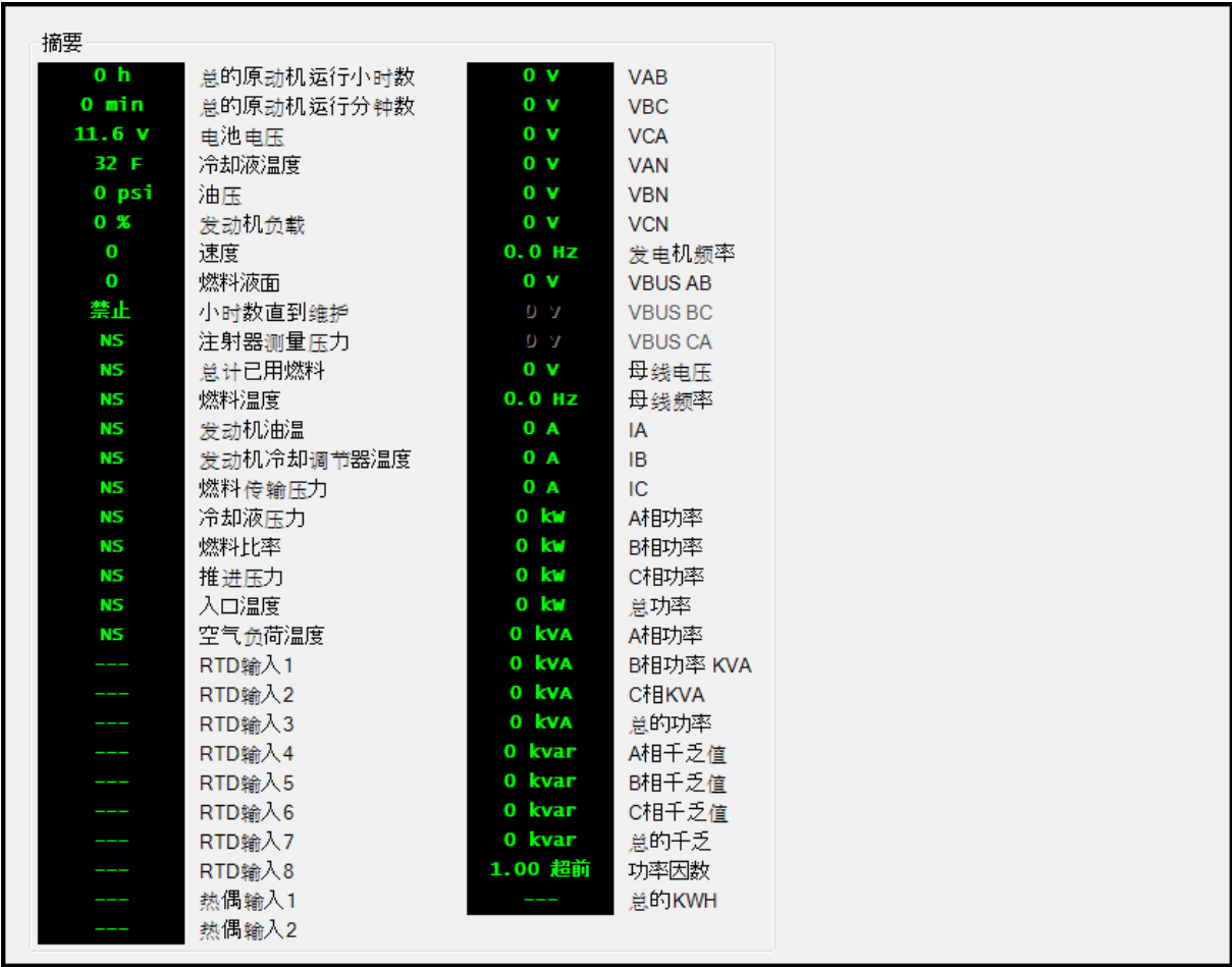
图 4-141. 测量，摘要
