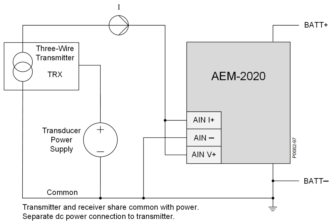
图 11-5. 模拟量输入 - 电流输入接线, III 型 2 线电路
