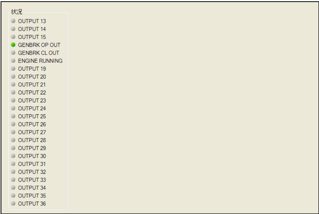
图 4-110. 测量，输出，输出触点
