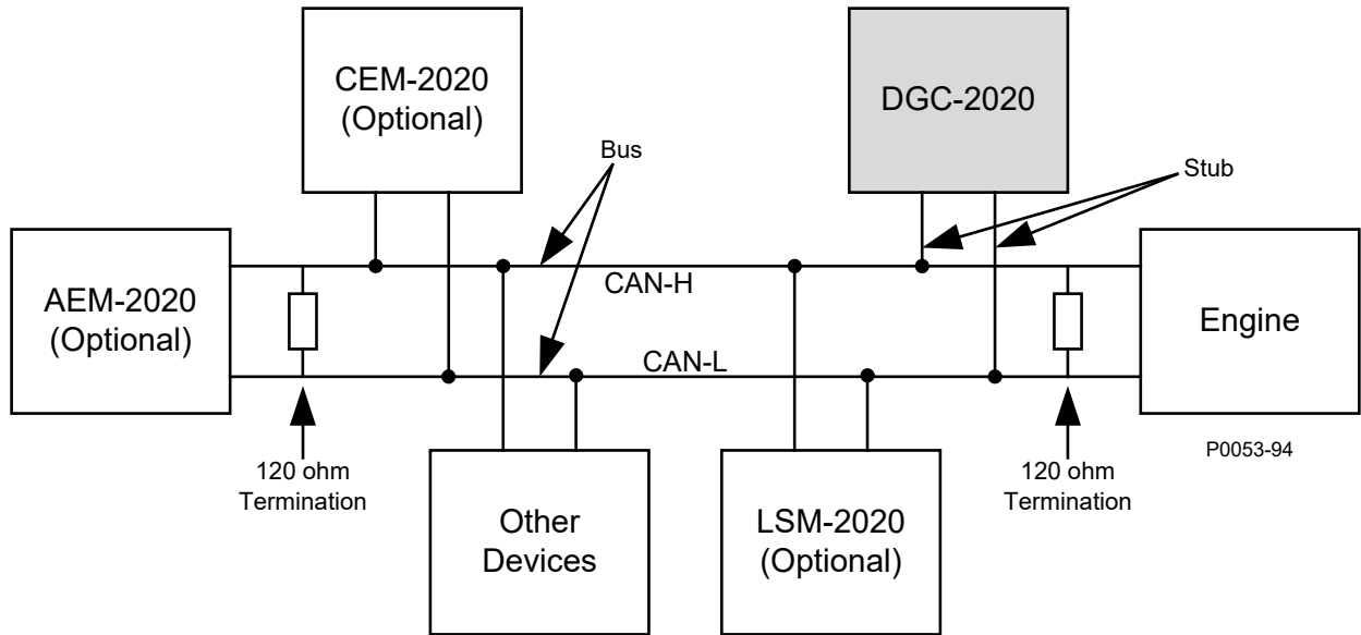
图 6-6. CAN Bus 接口, 可选 AEM-2020 作为母线一端
