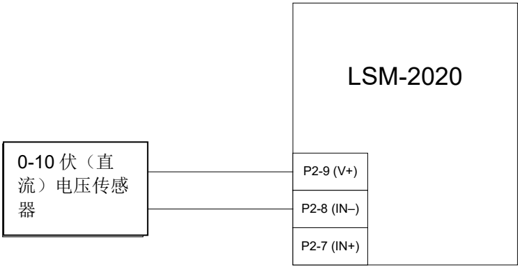
图 9-7. 模拟量输入 - 电压输入接线
