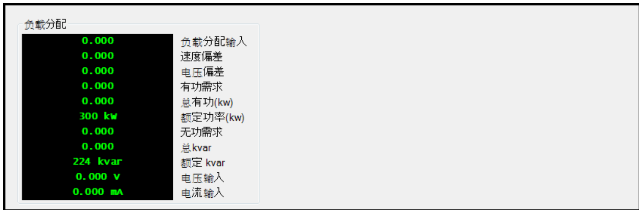
图 4-148. 计量探测器、诊断、负载分配界面
