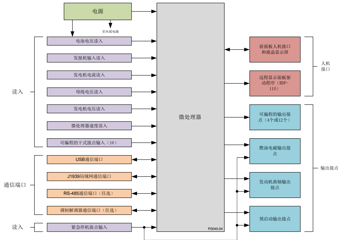
图 3-1. 功能块图表
