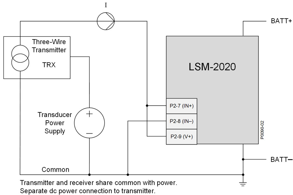
图 9-5. 模拟量输入 - 电流输入接线, III 型 2 线电路
