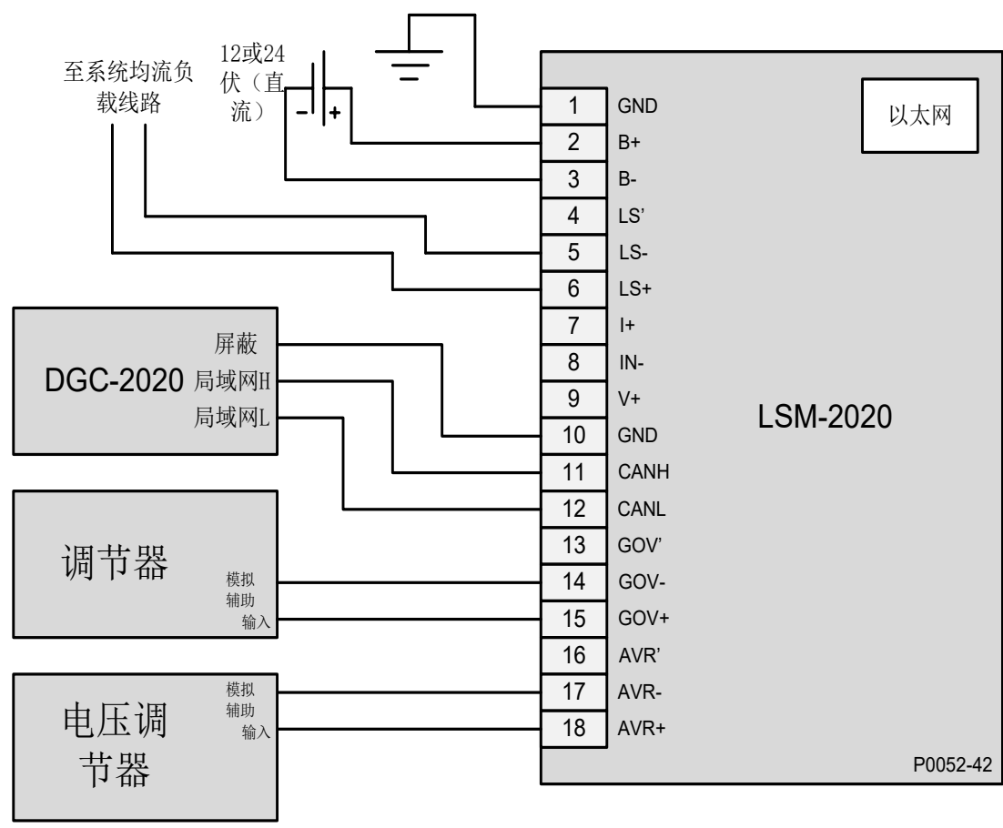
图 9-10. 典型 LSM-2020 接线
