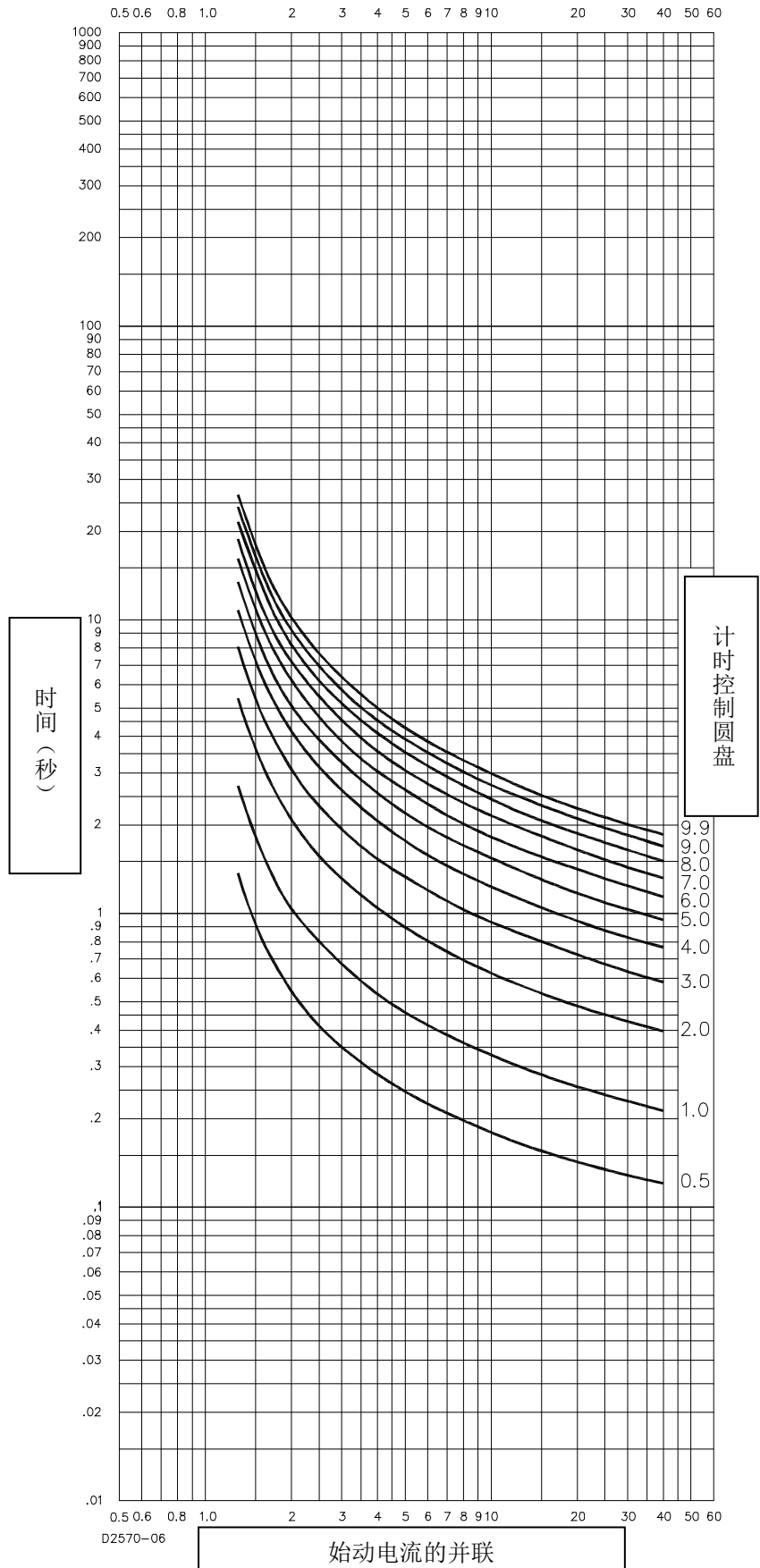
图 A-13. 时限特性曲线 A, 标准反时限 (BS 142)
