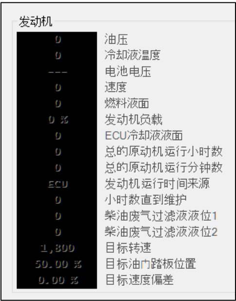
图 4-89. 测量，发动机
