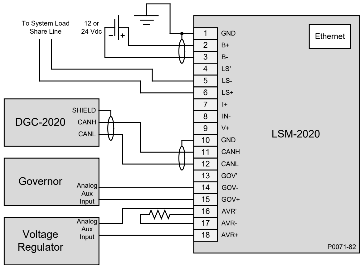
图 9-12. AVR, GOV 和 LS 端子的接线
