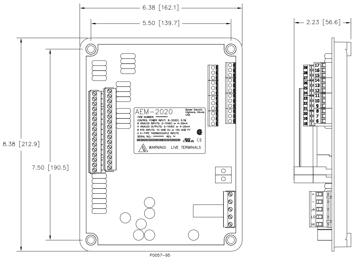
图 11-1. AEM-2020 总尺寸
